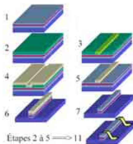
Les étapes de nanofabrication du dispositif de mesure d'une structure semi-conductrice en forme de nanofil.
